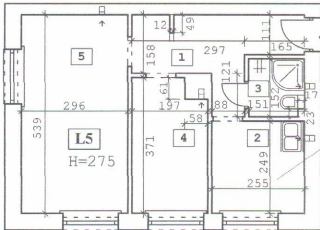
RZUT MIESZKANIA 1:100
