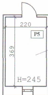
RZUT PIWNICY 1:100
