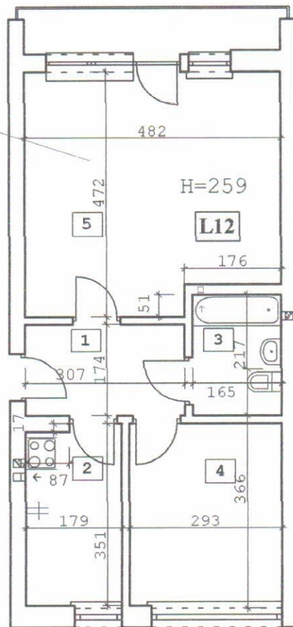
RZUT MIESZKANIA 1:100
