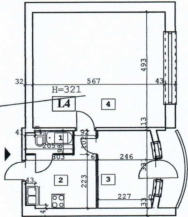
RZUT MIESZKANIA 1:100
